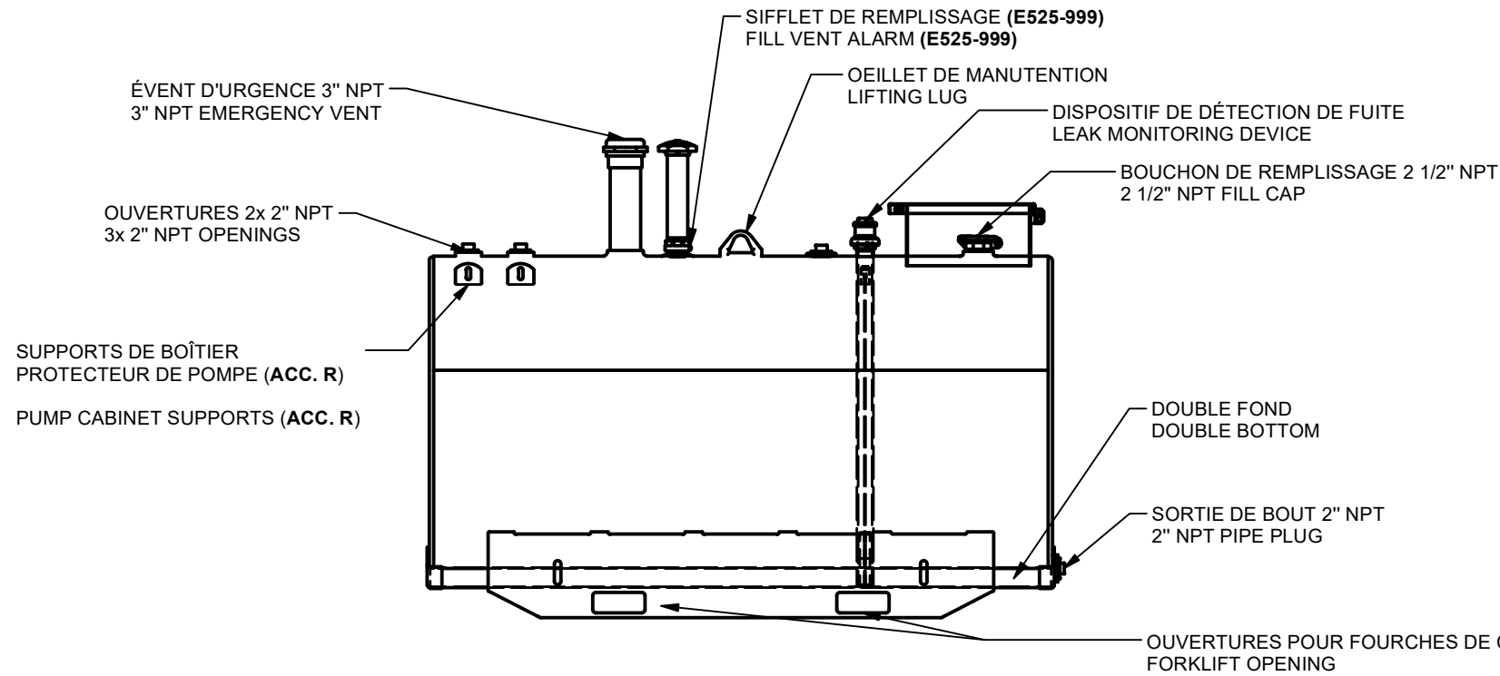
3014722 DOUBLE FOND / DOUBLE BOTTOM
